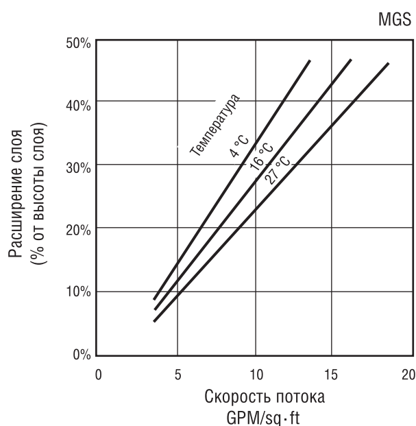
Рис. 2.9. Расширение слоя во время обратной промывки
